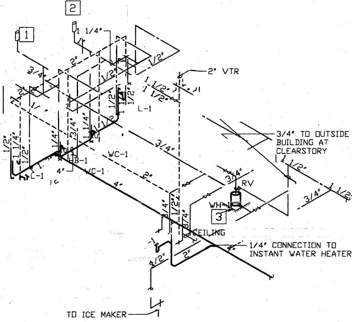
1 PLUMBING RISER M-2 SCALE: NONE
