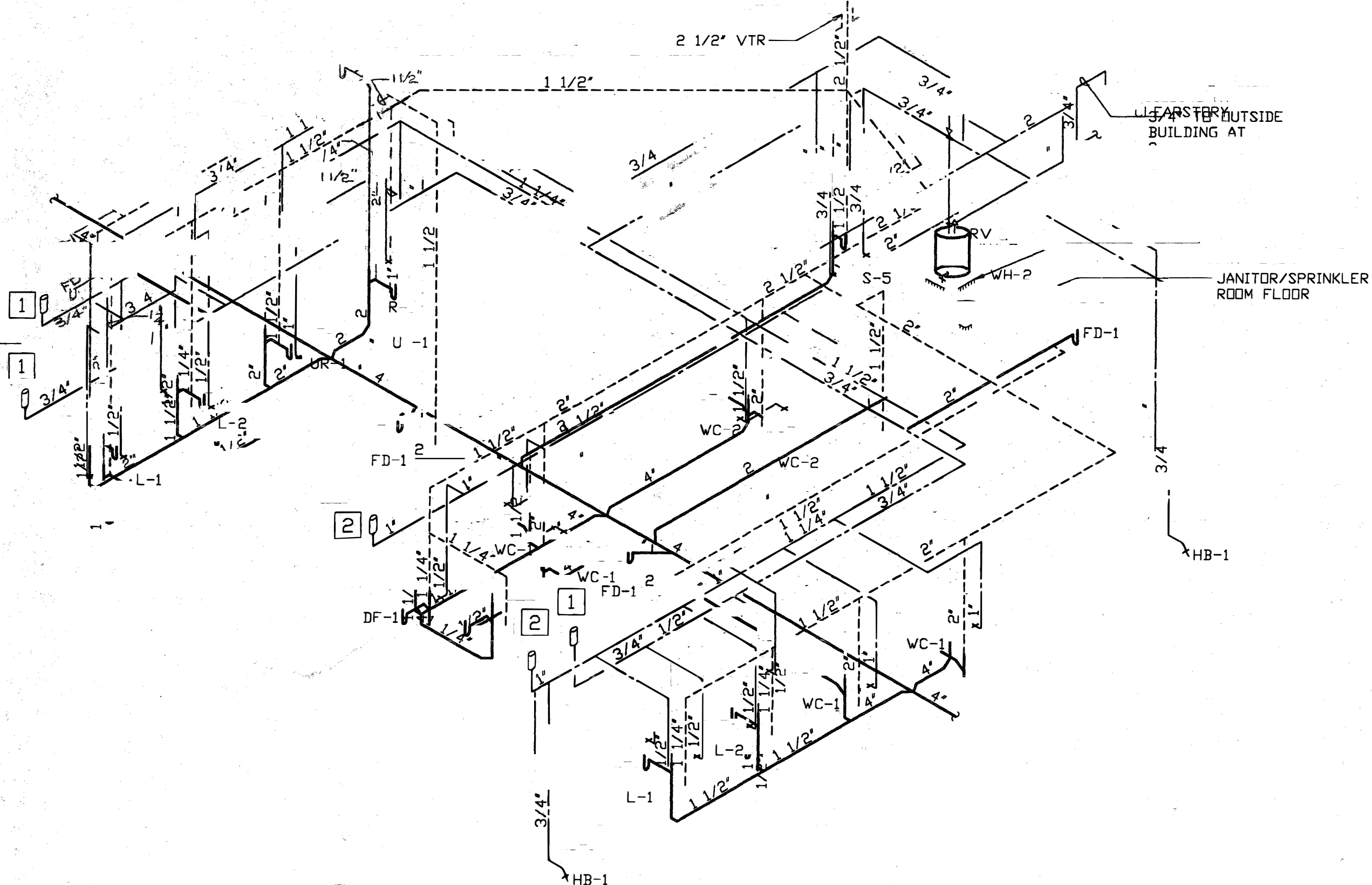
2 PLUMBING RISER M-2 SCALE: NONE
